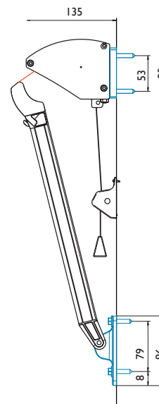
Väggmontering DA32 (mm).
